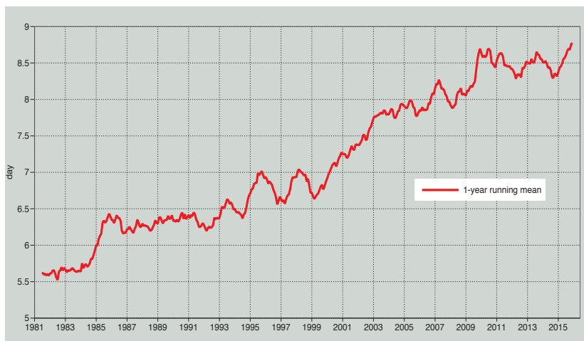
Evolution de la compétence prévisionnelle à moyenne échéance du CEPMMT au cours des 35 dernières années. La courbe indique le nombre de jours pendant lesquels les prévisions contiennent des informations utiles. Pour le définir, on prend le jour au-delà duquel, dans l'hémisphère Nord, la corrélation des anomalies à l'altitude géopotentielle 500 hPa chute sous le seuil de 60 %.
