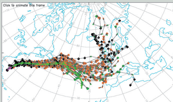
Figure 1. Trajectoires de Bertha dans les extratropiques, telles que prévues par les prévisions d'ensemble (lignes grises), la prévision de contrôle (ligne verte fine) et la prévision à résolution fine (HRES) (ligne verte épaisse). Bertha a touché l'Europe de l'Ouest aux alentours du sixième jour de la prévision.
