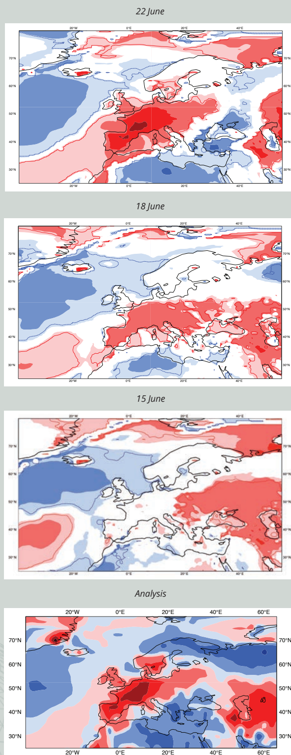
Figure 3. Prévisions de la température à 2 mètres : Anomalie hebdomadaire pour la période du 29 juin au 5 juillet tirée de l'analyse (en bas) et des prévisions des 22 juin (en haut), 18 juin (en dessous) et 15 juin (en dessous).
