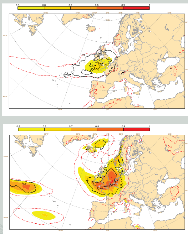
Figure 2. Indice de prévision d'événements extrêmes (EFI) de vitesse du vent pour la période du 10 au 12 août 2014, à des échéances de 6 à 9 jours (haut) et à 2 à 5 jours (bas).
