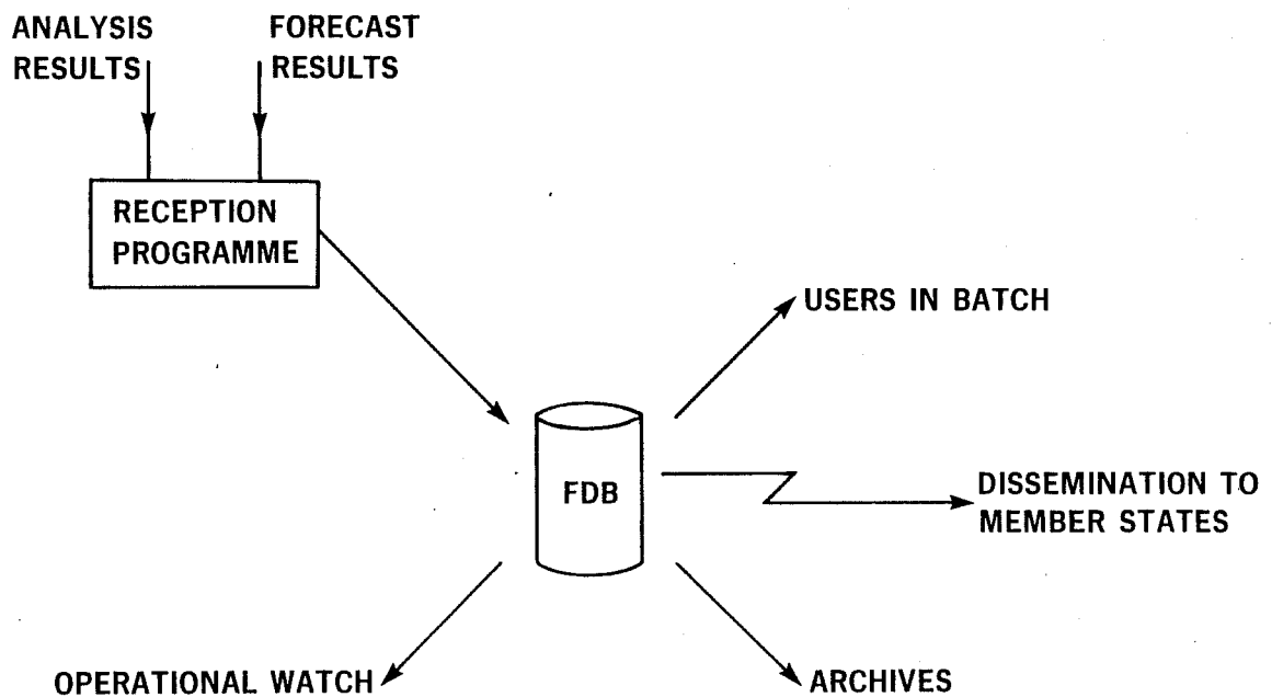
Fig. 5 Processes using FDB
