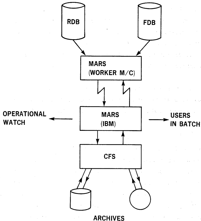
Fig. 7 The MARS Archive/Retrieval
